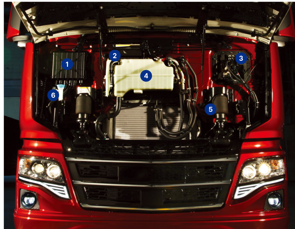
① 멀티 커넥터 ② 에어컨 필터 ③ 브레이크 페달 모듈 ④ 냉각수 탱크 (서지탱크) ⑤ 전방 캡 서스펜션 ⑥ 워셔액 주입구
